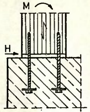
Stützenfuß (eingespannt)
