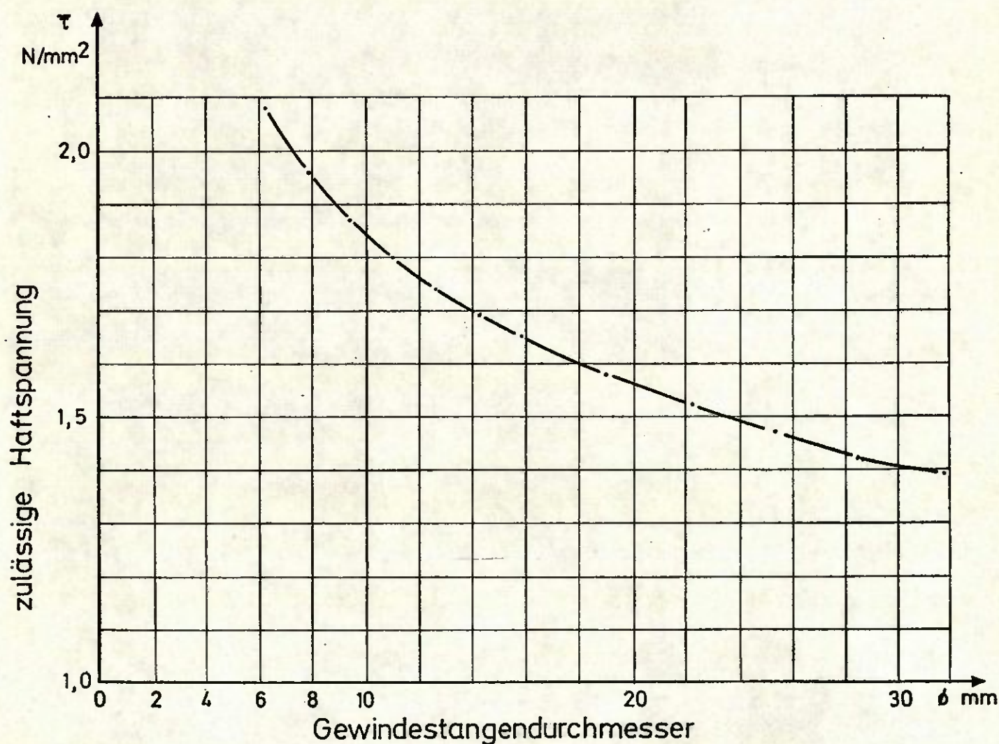
Bild 2: Zulässige Haftspannung für ohne Leim in Douglas-fir bzw. Lärche eingedrehte Gewindestangen nach "Timber Construction Manual" (Rohdichte = 0,51 \text{ g/cm}^3 )
