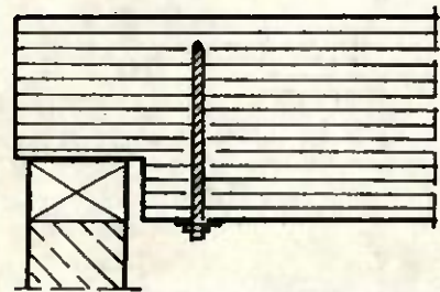
Träger- Ausklantung
