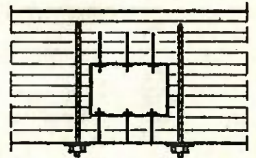
Träger- Durchbruch
