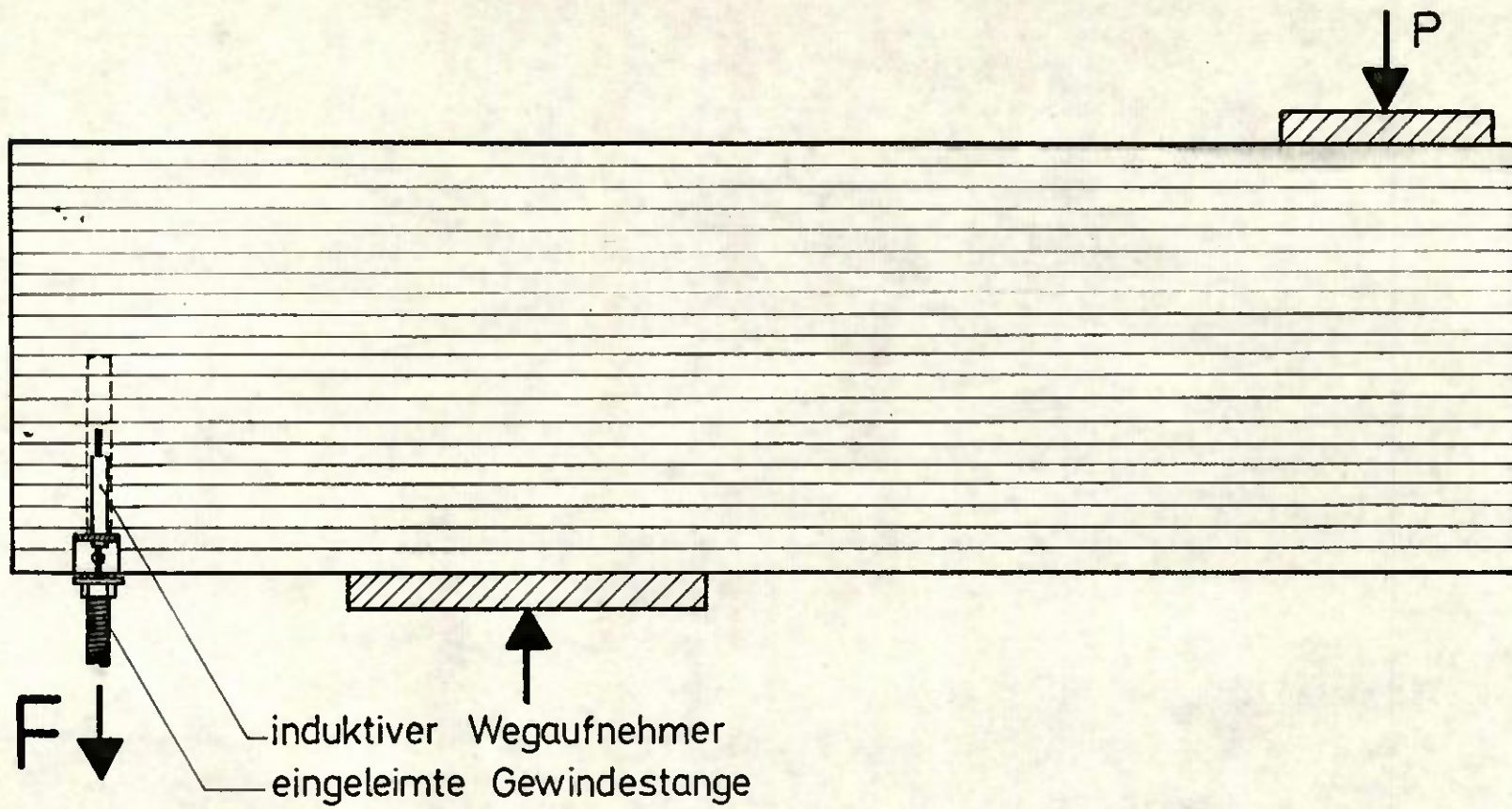
Bild 9: Versuchsaufbau und Anordnung der Meßvorrichtung bei Prüfkörpern der Versuchsreihe SA
