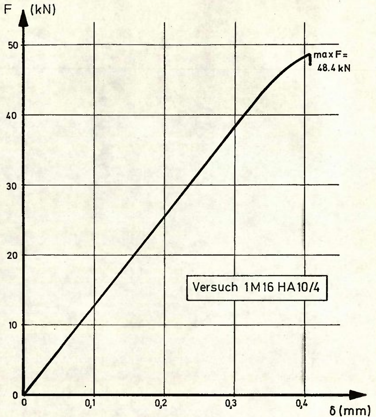
Bild 11: Last-Verformungs-Diagramm des Prüfkörpers 1M16HA10/4
