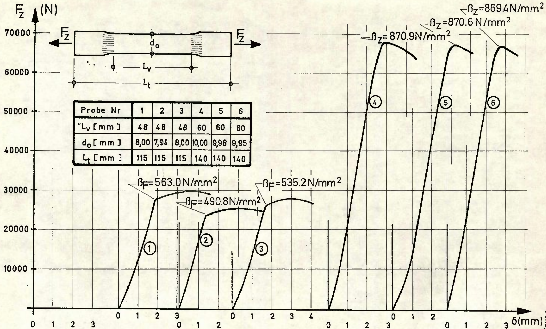
Bild 16: Zugversuche an Stahlproben nach DIN 50125
