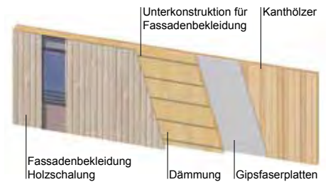
Blockständer-Elemente als Außenwände (im Werk vorgefertigt einschließlich Fenster und fertiger Fassadenbekleidung)
