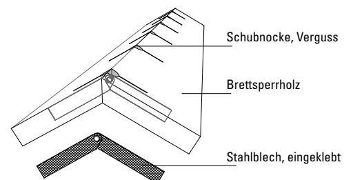
Holzplattenverbund mit Schubnocken
