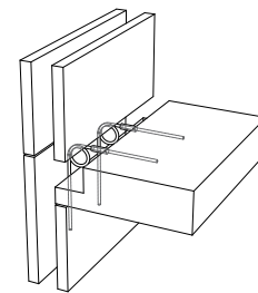
Rahmenartiges Endauflager, Beton - Holzdecke
