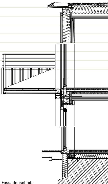
Fassadenschnitt
