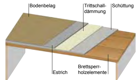
Brettsperrholzelemente als Decken
