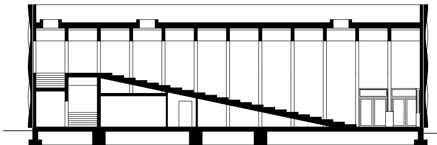
Längsschnitt
