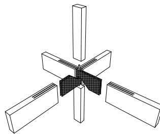
Kreuzverbinder mit Verguss
