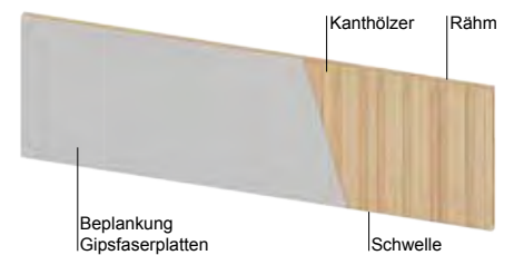
Blockständer-Elemente als Innenwände
