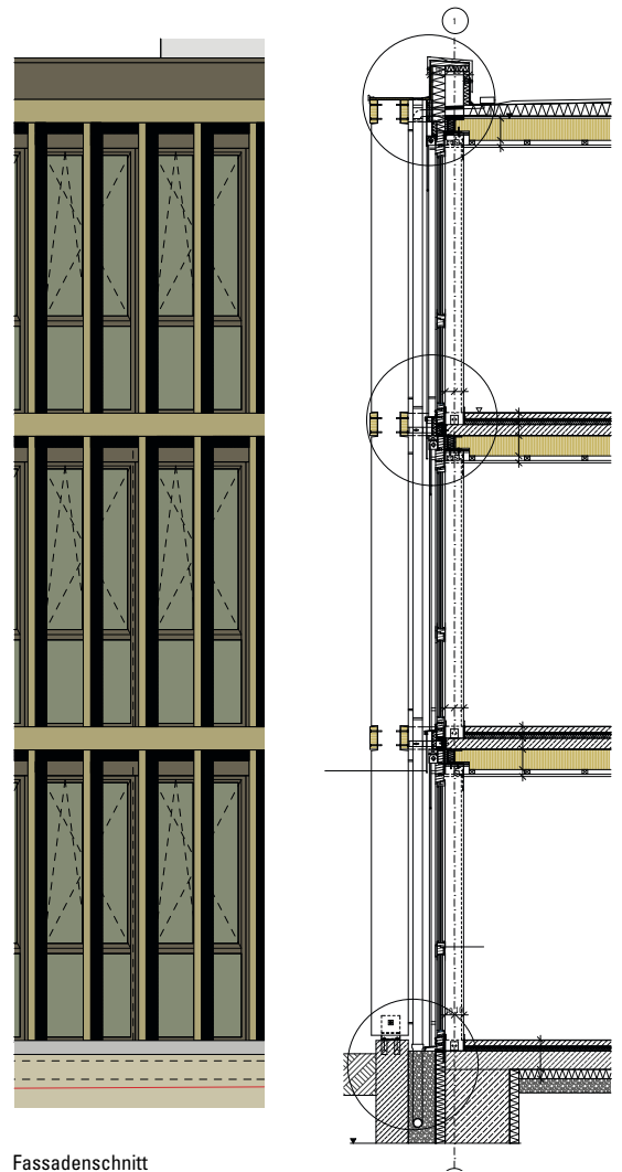
Fassadenschnitt
