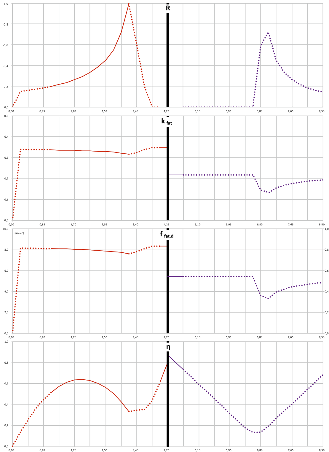
Bild 6.3: Schrittweise Durchführung des Ermüdungsnachweises beim 2-Feld-Träger
