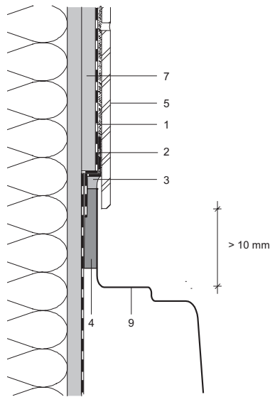
Abb. 6.4-2 Beispiel: Anschluss Duschtasse – Wand mit hochgezogenem Duschtassenrand
