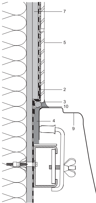
Abb. 6.4-1 Beispiel: Befestigung von Sanitäröbekten mit Wannenleisten
