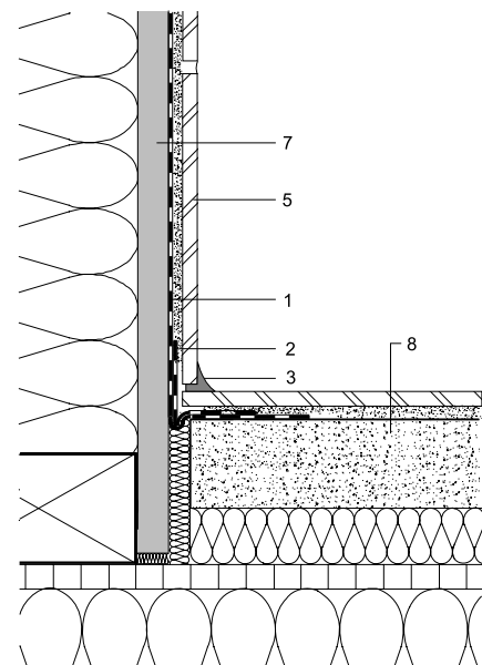
Abb. 6.3-3 Beispiel: Boden-Wand-Anschluss
