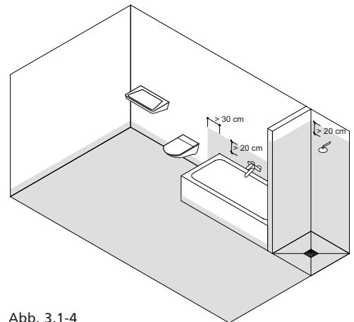
Abb. 3.1-4 Häusliches Bad mit Wanne ohne Duschnutzung und planmäßig genutztem Bodenablauf im Duschenbereich
