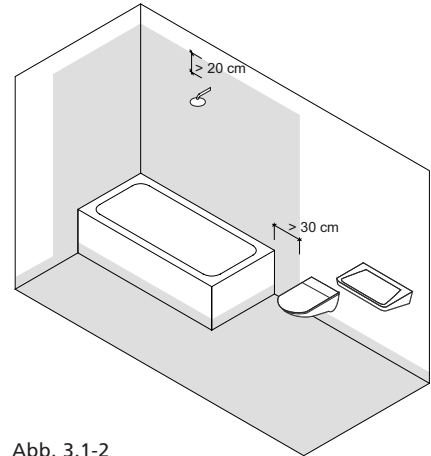
Abb. 3.1-2 Häusliches Bad mit Badewanne als Dusche
